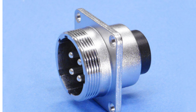
写真はシェルサイズ 24 RM (圧着Cタイプ)
